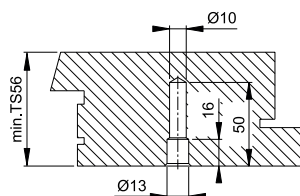
Holz-Profil
